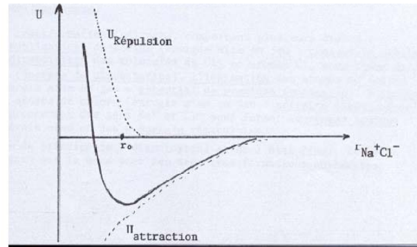
L'énergie potentielle d'interaction ionique en fonction de la distance entre les 2 ions
